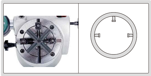
沟槽测头测量小尺寸内径与内沟槽直径
