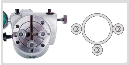
盘形测头测量外径
