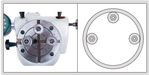
盘形测头测量大尺寸内径
